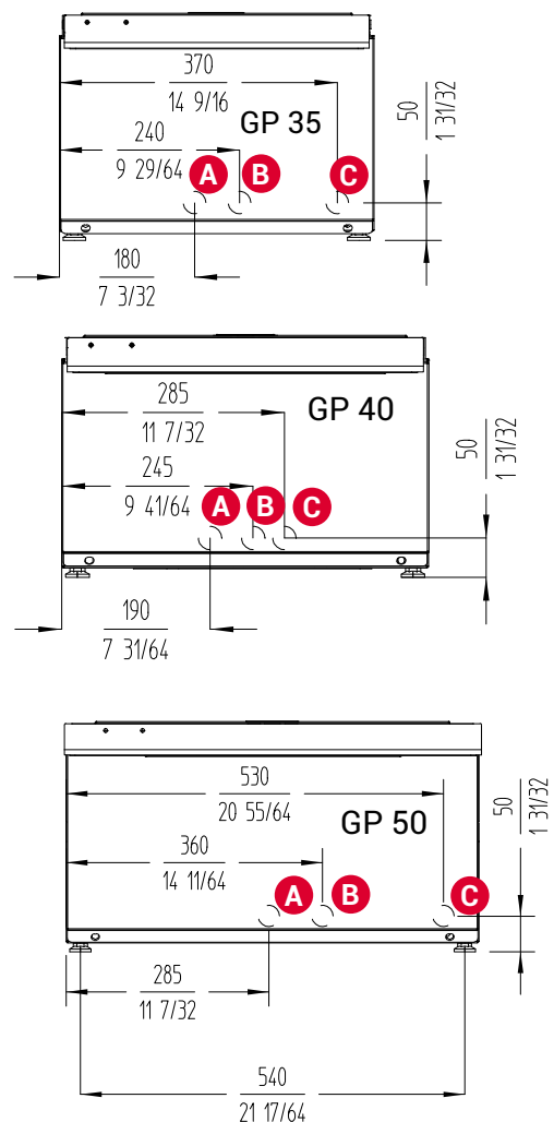
Abb. 1: Maschinenanschlusspunkte
